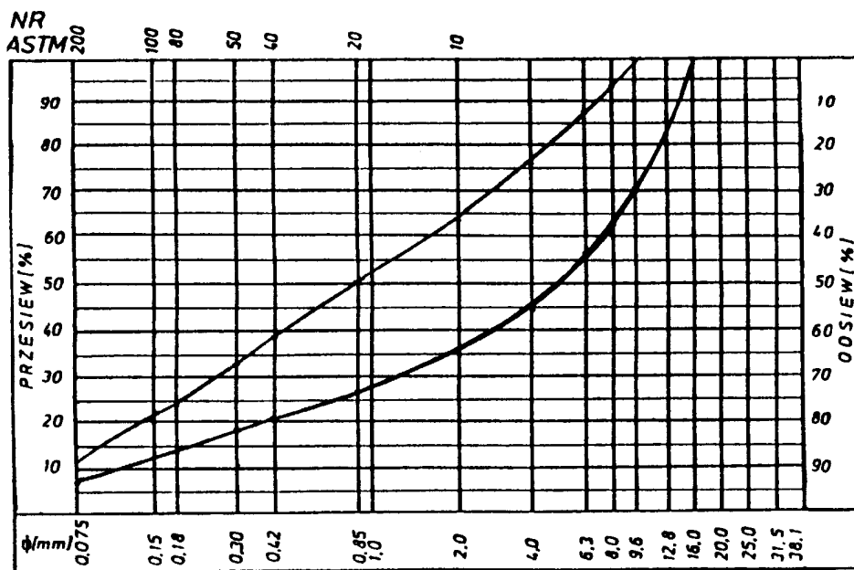
Rys. 1. Krzywe graniczne uziarnienia mieszanki mineralnej BA od 0 do 16mm, od 0 do 12,8 do warstwy ścieralnej nawierzchni drogi o obciążeniu ruchem KR1 lub KR2
